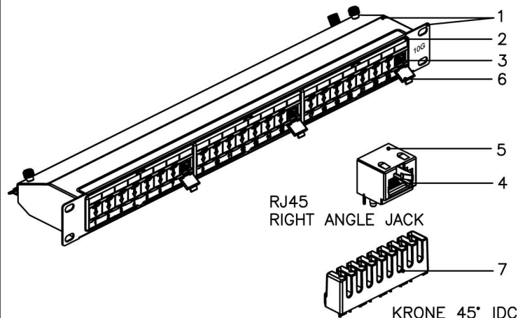
KRONE 45° IDC
